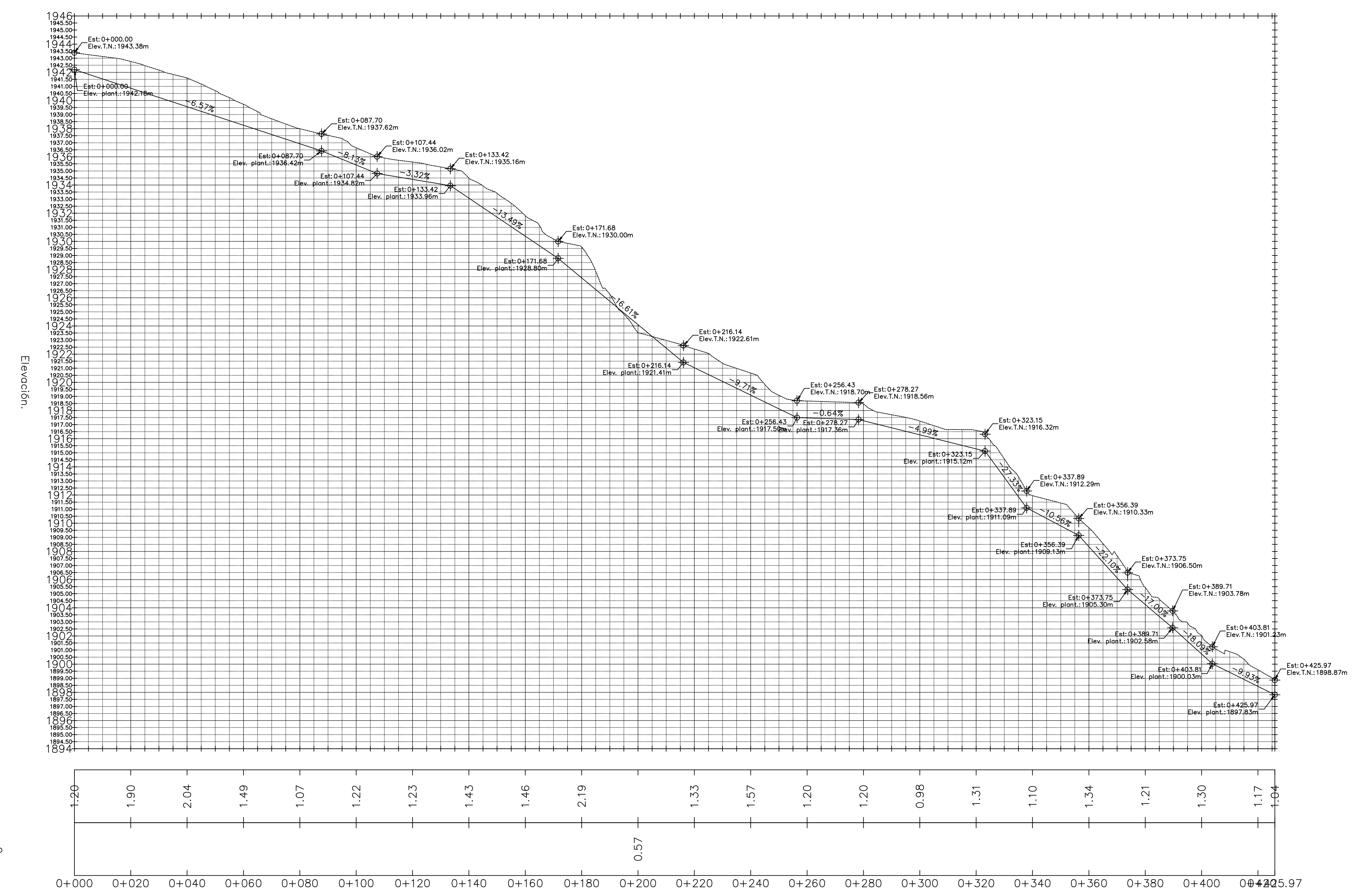
Perfil drenaje sanitario
